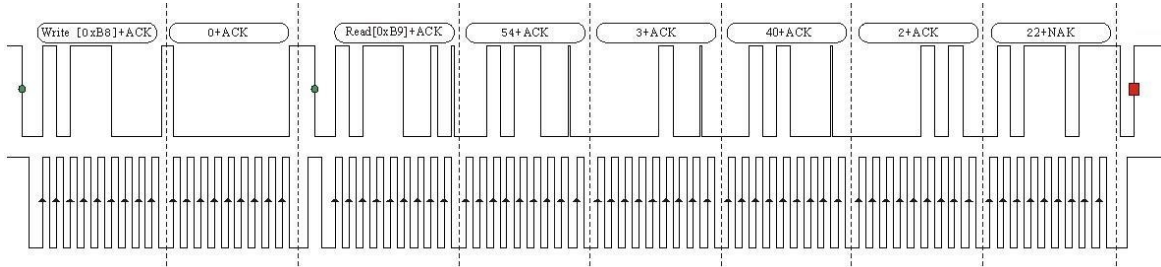
图 15 Reference sequence diagramNote: the actual test data
