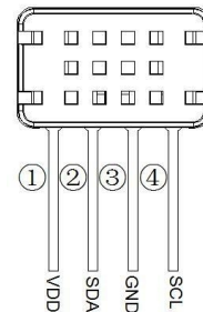
图 4 : DHT12Wiring diagram
