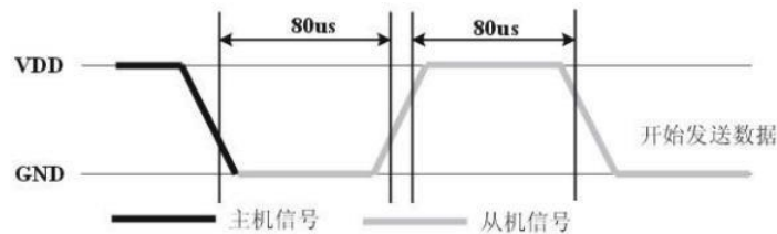
图 17 Signal
